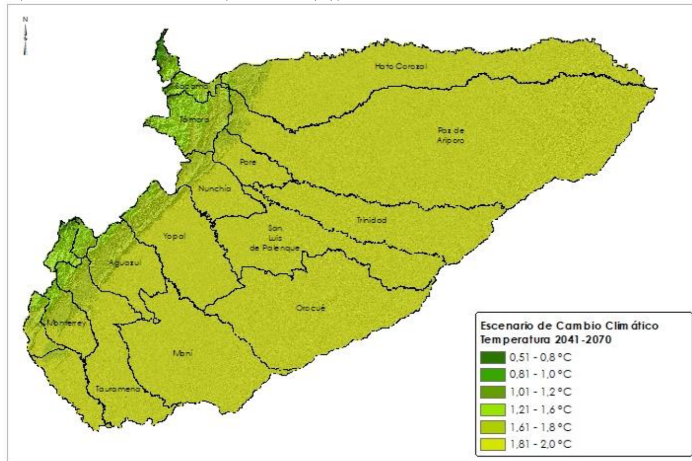
Mapa 21. Escenario de Diferencia de Temperatura Media (°C) para el 2041 - 2070 Vs 1976-2005
