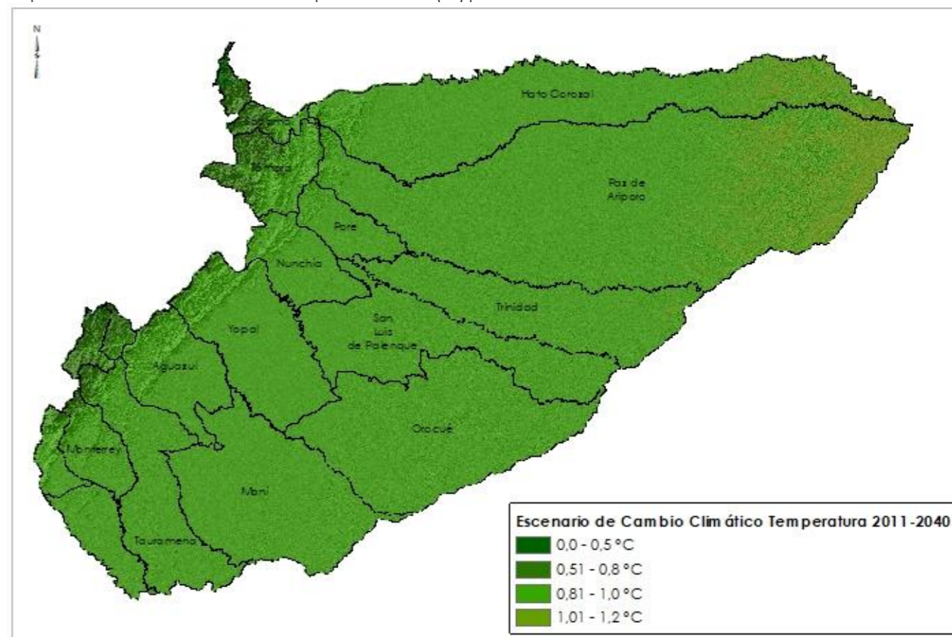
Mapa 20. Escenario de Diferencia de Temperatura Media (°C) para el 2011 - 2040 Vs 1976-2005
