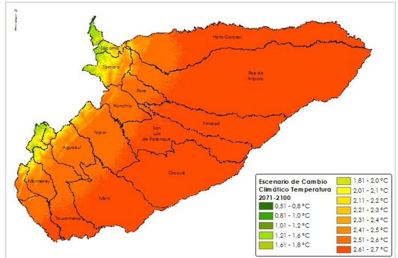
Mapa 22. Escenario de Diferencia de Temperatura Media (°C) para el 2071 - 2100 Vs 1976-2005
