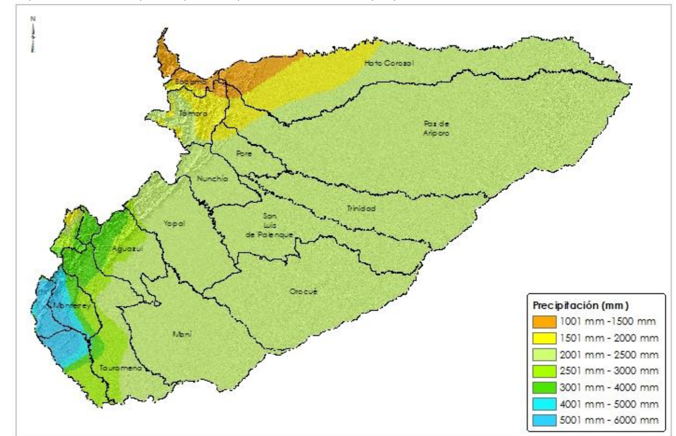
Mapa 15. Escenario Precipitación para el Departamento de Casanare (mm) Periodo 1976-2005
