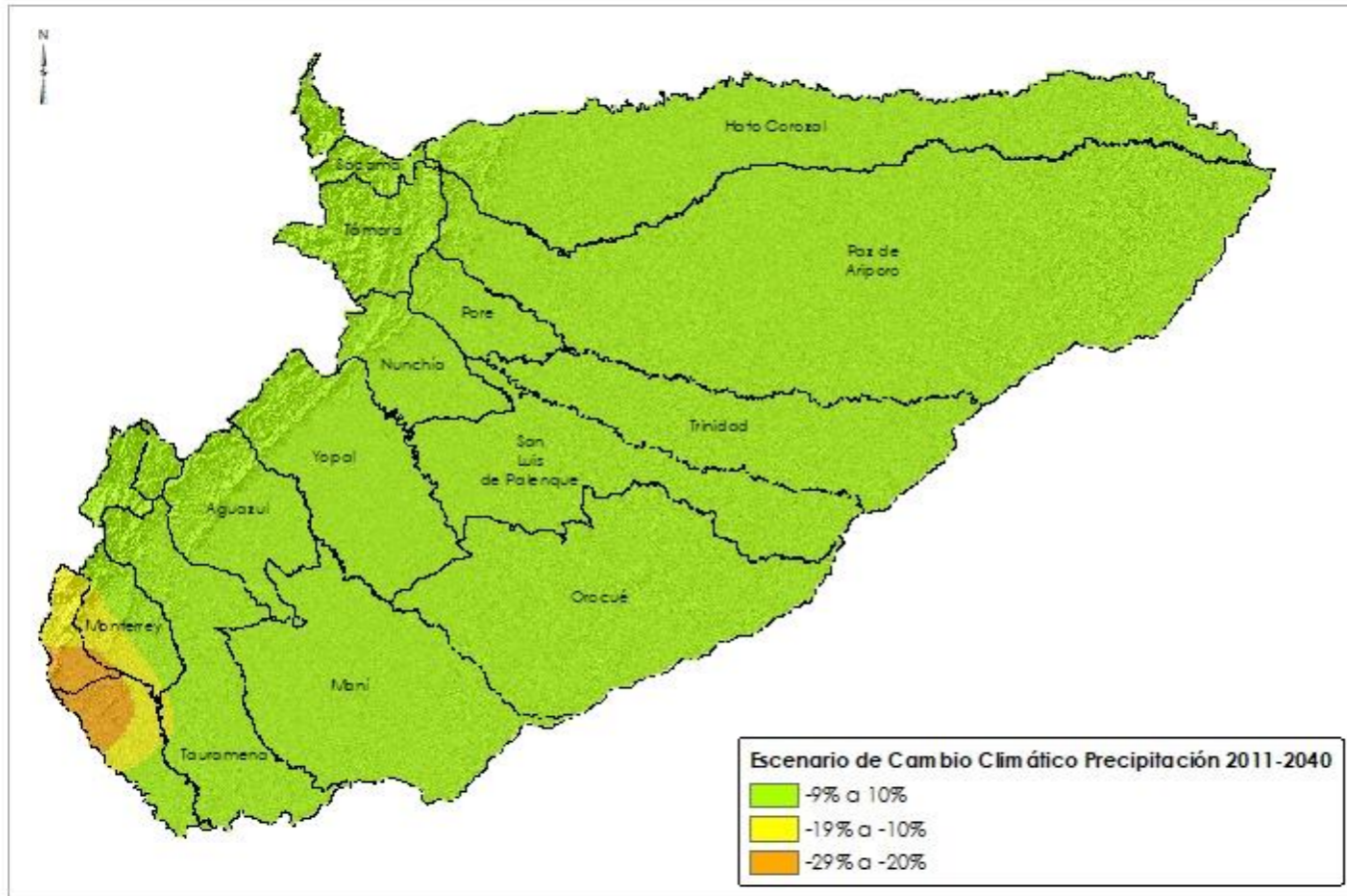
Mapa 16. Escenario Precipitación Ensamble Multiescenario 2011 - 2040 Vs 1976-2005
